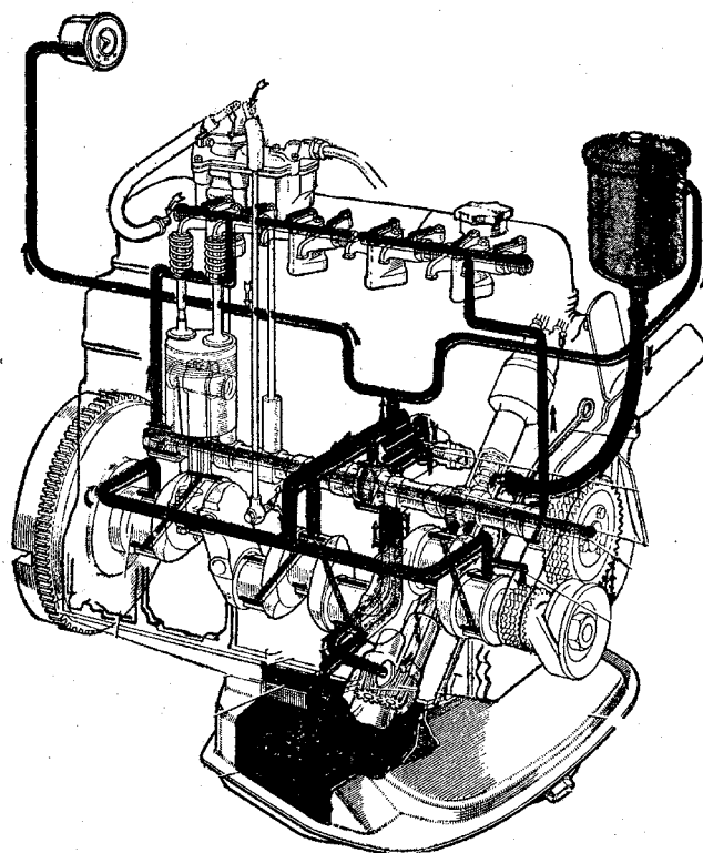
Lubricación a presión en un motor con válvulas a la cabeza
