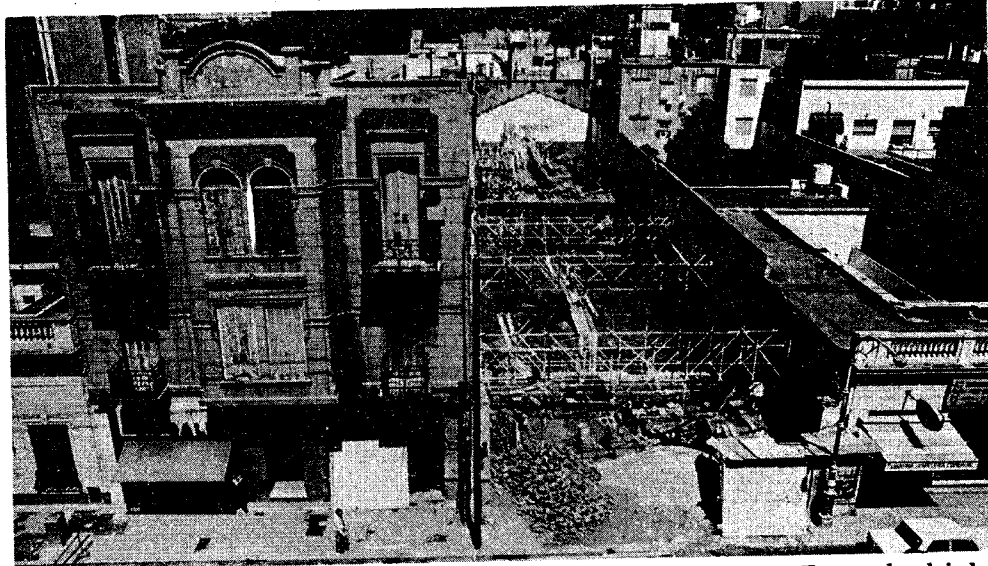
Los edificios ubicados a ambos lados de la excavación presentan rajaduras. Fueron desalojados.
