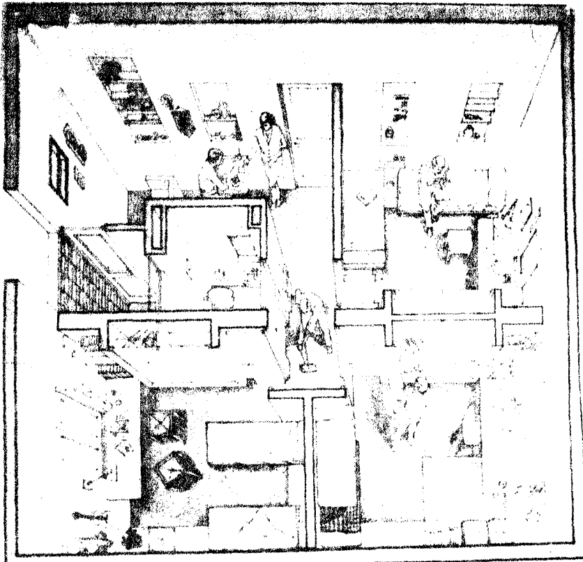
PERSPECTIVA Y DETALLE DE AMOBLAMIENTO EN UN DEPARTAMENTO DE LA RESIDENCIA
