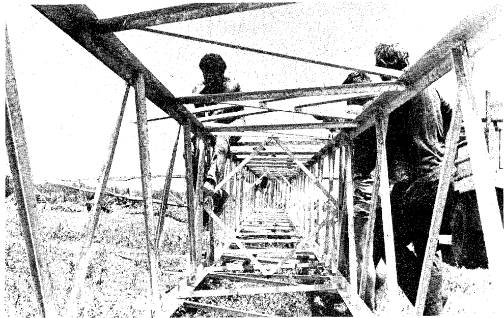
Los obreros de Hidronor y del Consorcio británico preparan la torre caída para que sea izada.
