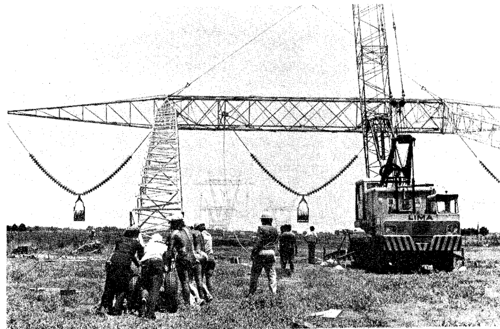
Montada sobre ruedas, la torre es conducida hasta la grúa con la cual se la elevará.
