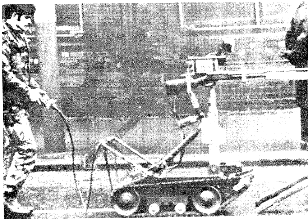
BELFAST. Un soldado inglés opera un robot electrónico de control remoto, equipado con un fusil, que lleva una cámara de TV conectada a un circuito cerrado. Los técnicos, desde distancia, pueden detectar donde hay una bomba y accionar el fusil sin poner en peligro su vida, destruyendo los explosivos. No obstante tantas precauciones, siguen explotando bombas en Irlanda. (Radiofoto de AP).
