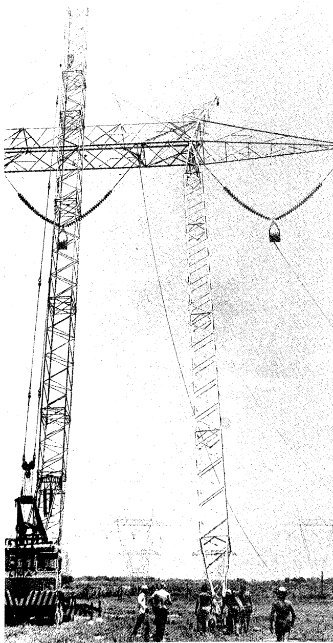
La tarea está por concluir y la torre recupera su verticalidad.
