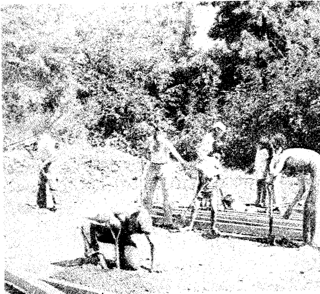
Construyendo un tinglado para una cooperativa de vivienda
