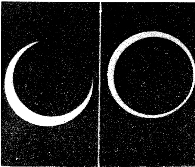
Secuencia del eclipse anular de sol registrada anteayer desde la localidad de Guanacaste, Costa Rica. Como se ve, hasta el sol fue víctima de un apagón en la jornada de Nochebuena.
