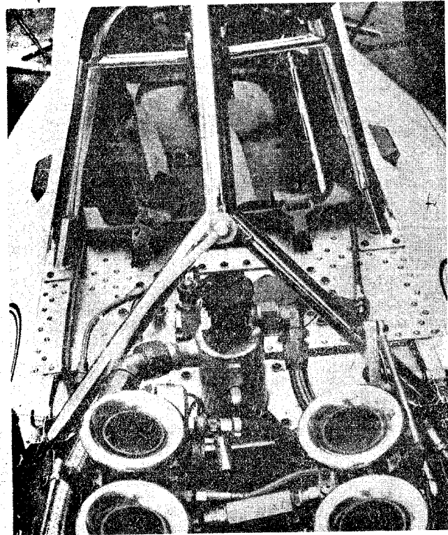
Robusta barra protectora para casos de vuelco. (Brabham BT 44)
